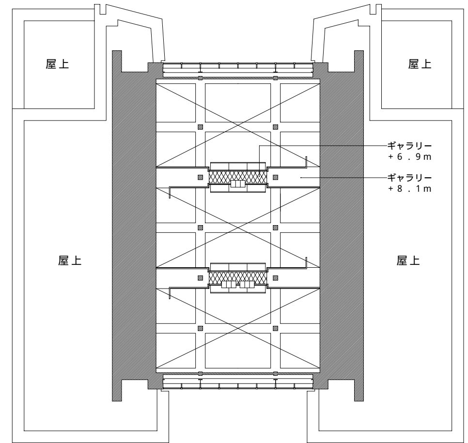
第2ギャラリー平面図
