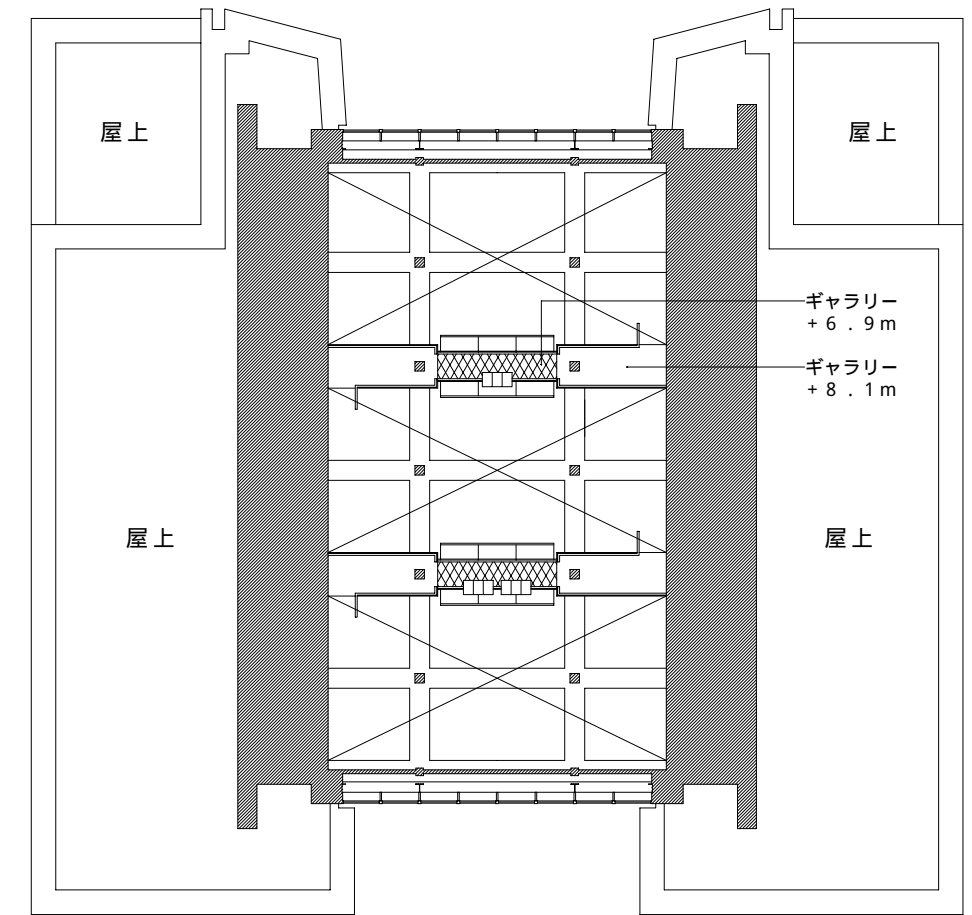
第2ギャラリー平面図
