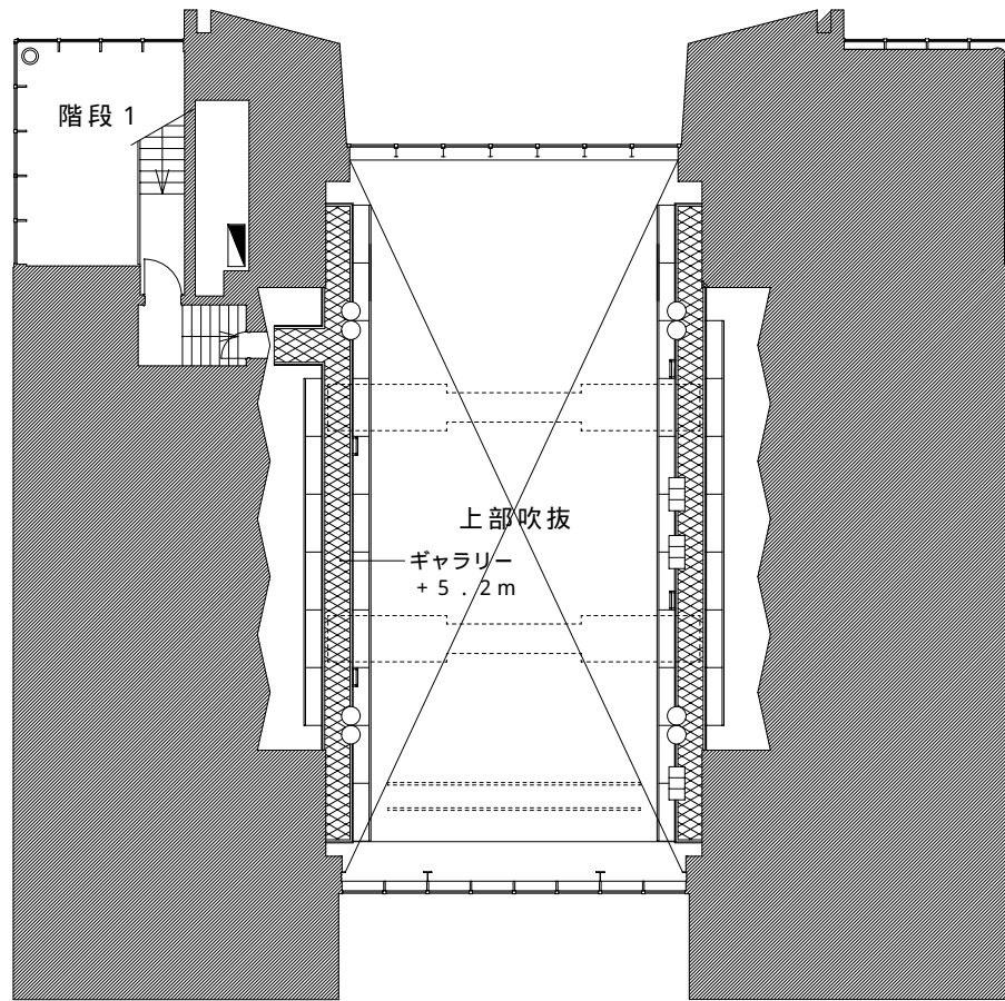
第1ギャラリー平面図
