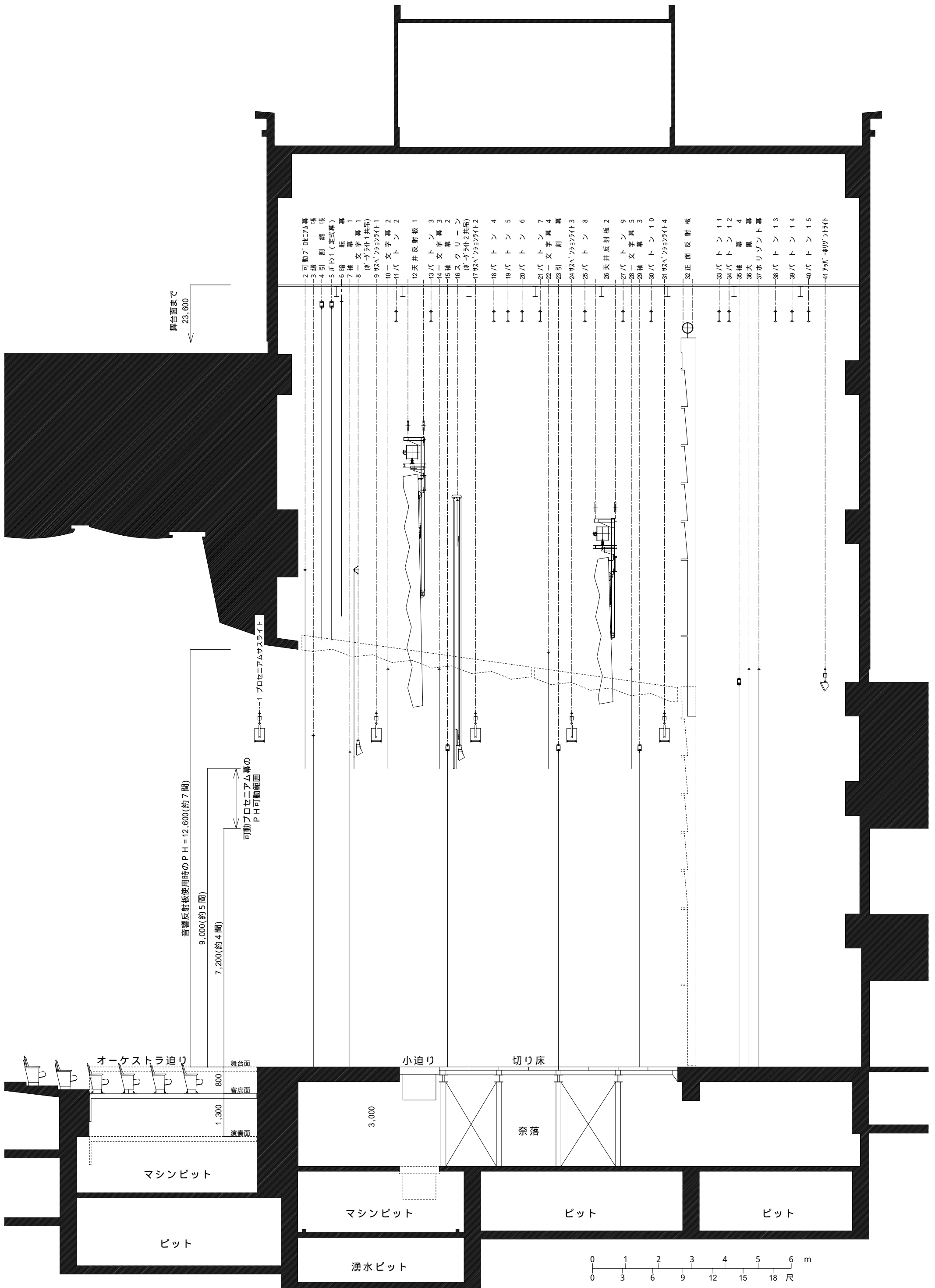
酒田市民会館「希望ホール」 舞台断面図 ( 1 / 100 )
